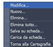
Menu Rotte
