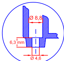
Hole/Foro Ø 4,6 mm
