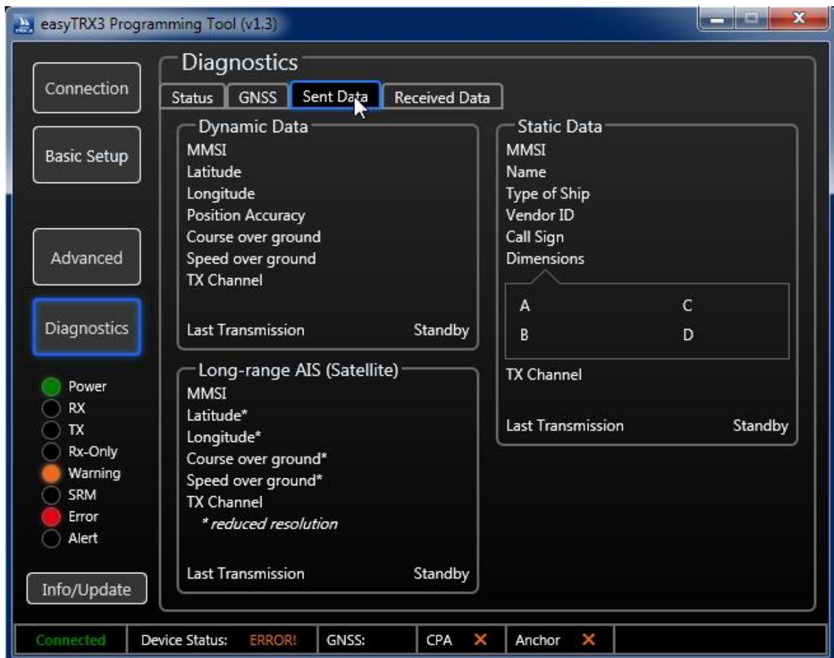
Abbildung 47 Anzeige Send-Data
