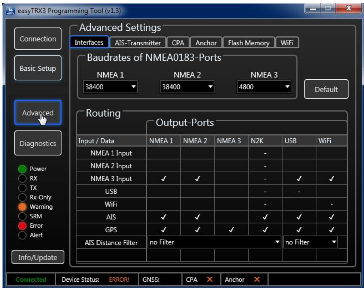
Abbildung 17 Eingabefenster Data-Routing
