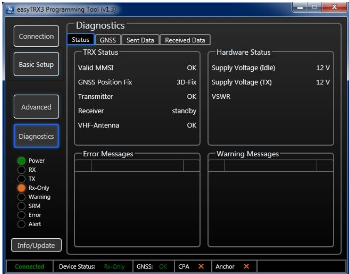
Abbildung 44 Diagnose-Fenster
