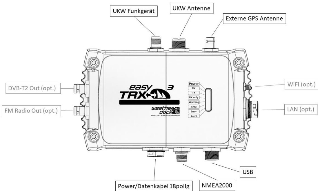
Abbildung 2 Anschlüsse
