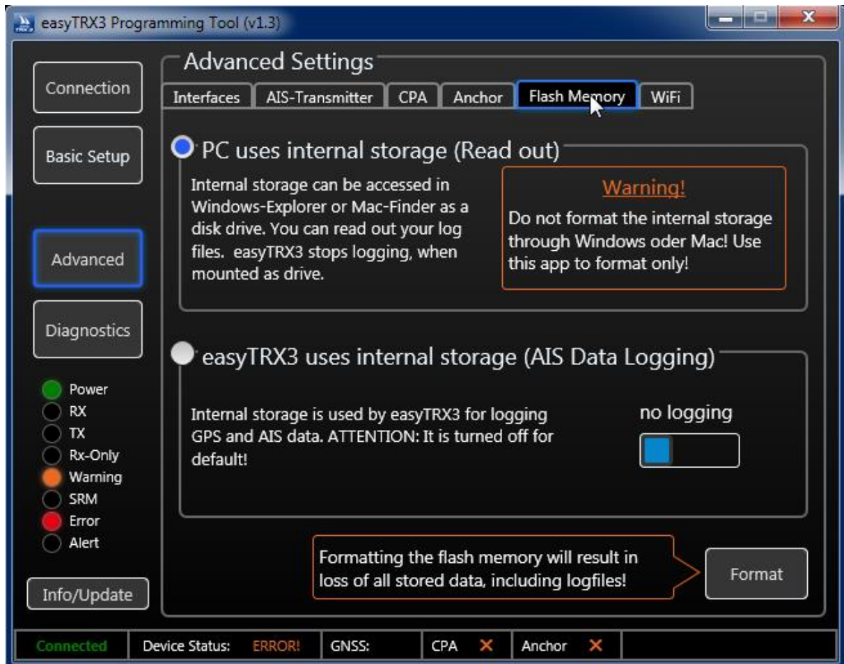
Abbildung 28 Einstellungen Flash-Memory
