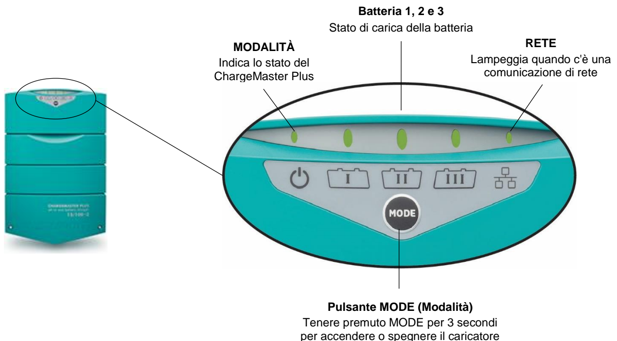
Figura 5: ChargeMaster Plus Display di stato
