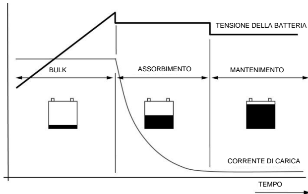
Figura 6: processo di carica
