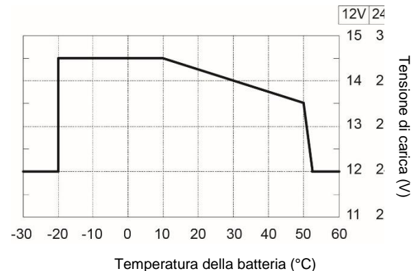
Figura 7: Carica con compensazione di temperatura
