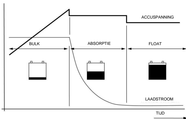
Afbeelding 6: laadproces
