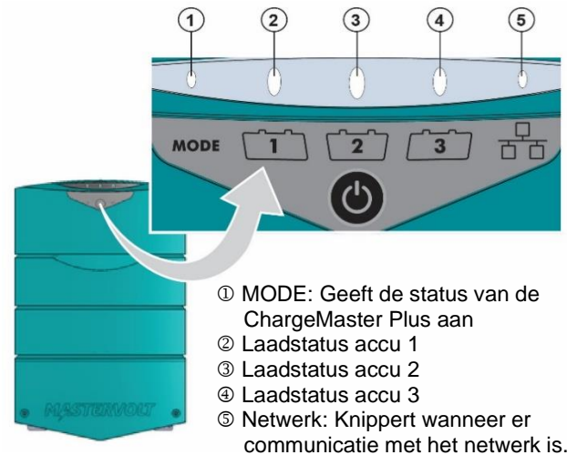
Afbeelding 5: ChargeMaster Plus statusdisplay
