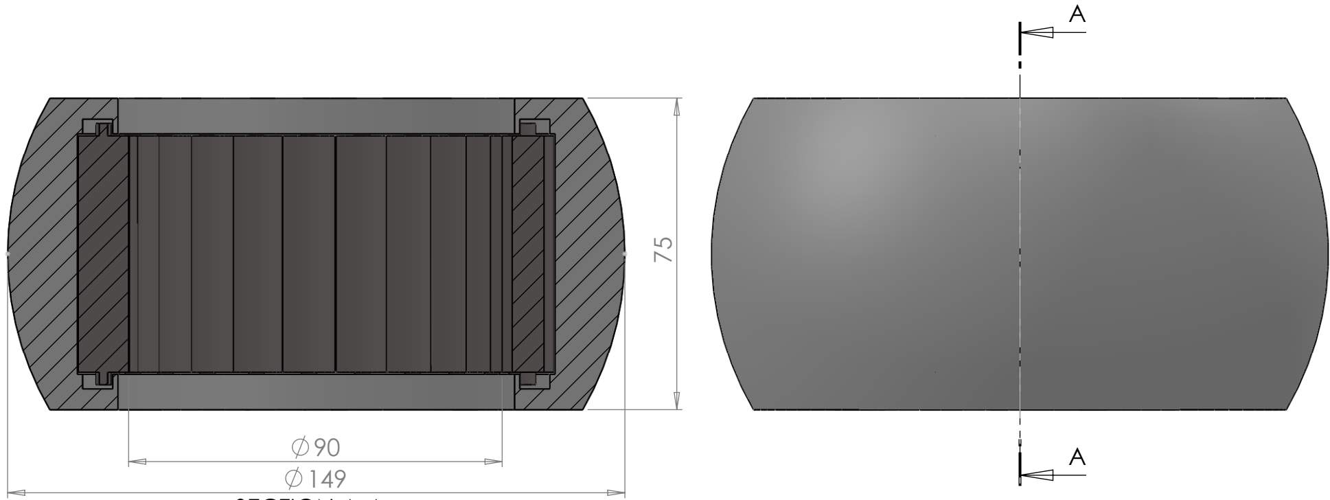
SECTION A-A SCALE 1 : 1.25
