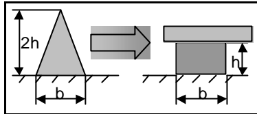
Afbeelding 1: Aanbrengen driehoeksruips
