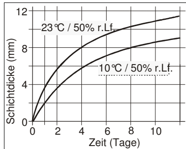
Diagramm 1: Durchhärtageschwindigkeit für Sikaflex®-252
